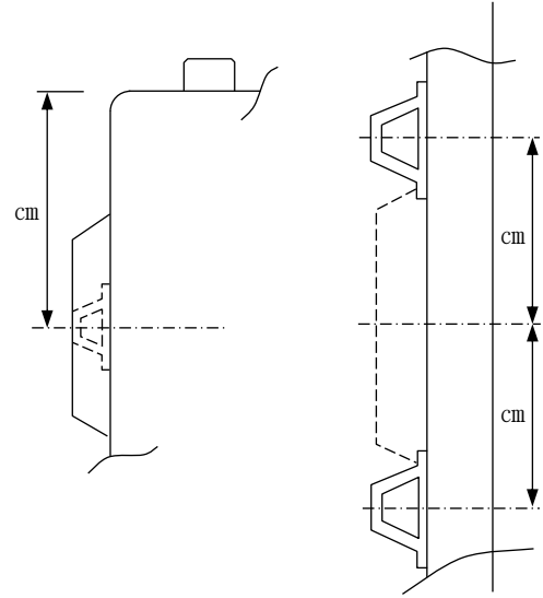
防眩材測定位置
