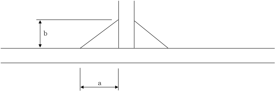
突合わせ溶接出来形管理表
