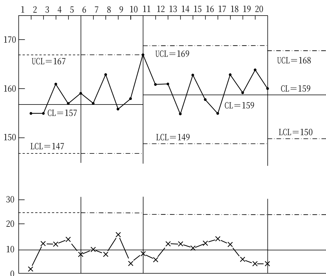
図-13 \bar{\chi}-R 管理図
