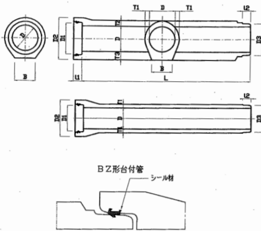
BZ 形台付管：管の受け口に予めシール材が埋込まれた構造（ガスケットタイプ）
