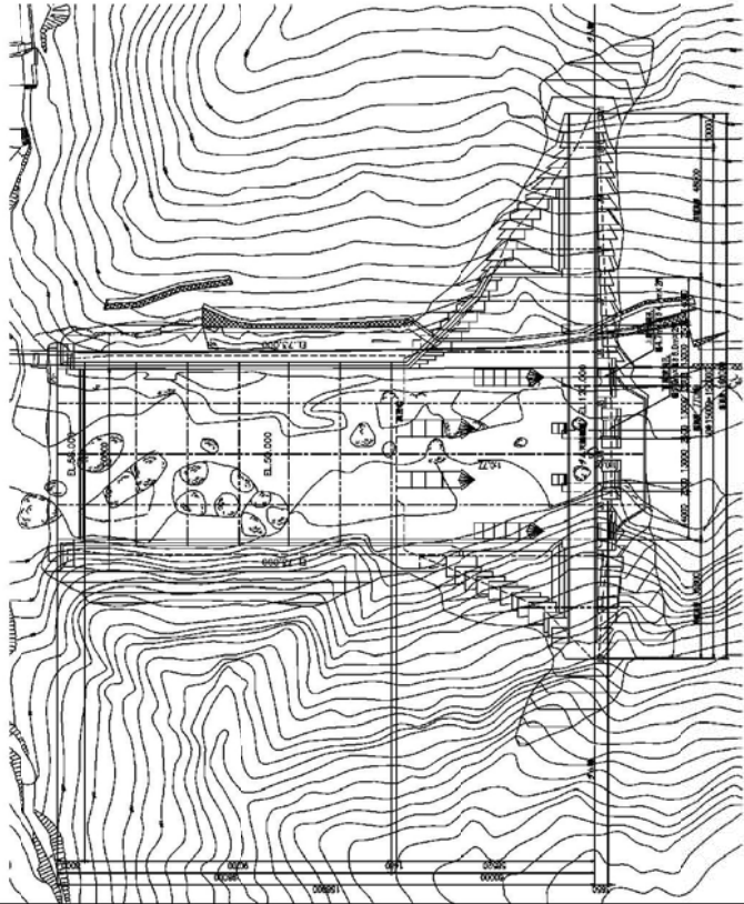
平面図
